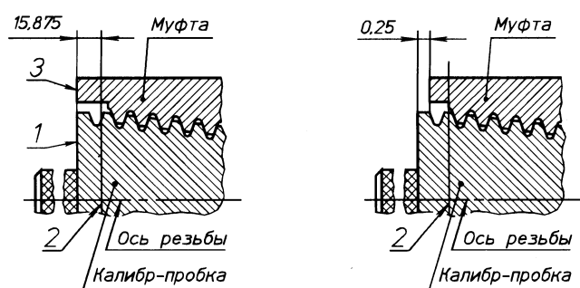
1 — контрольная плоскость; 2 — основная плоскость; 3 — упорный торец
