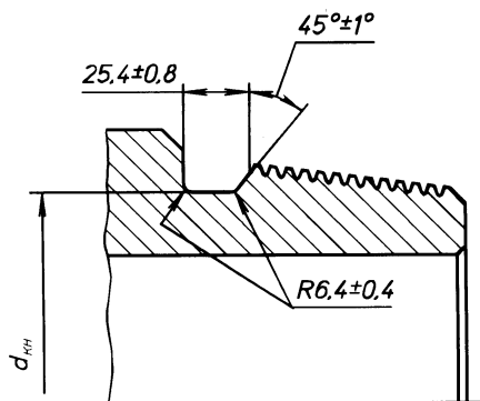
Рисунок В.1 — Разгрузочная канавка ниппеля
